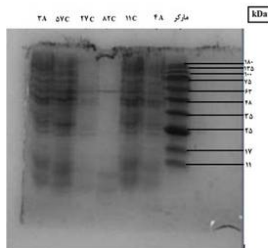
تصویر ۲: الگوی پروتئینی جدایه‌های یرسینیا راکری به دست
