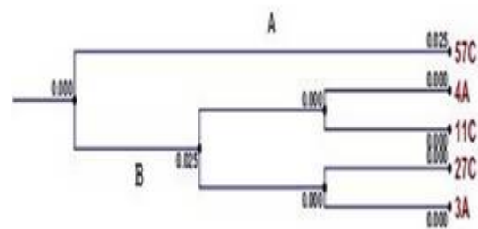
شکل ۴: درخت فیلوژنی حاصل از الگوی پروتئینی جدایه‌های یرسینیا راکری به دست آمده از مزارع قزل‌آلای کشور با استفاده از نرم‌افزار UPGMA
