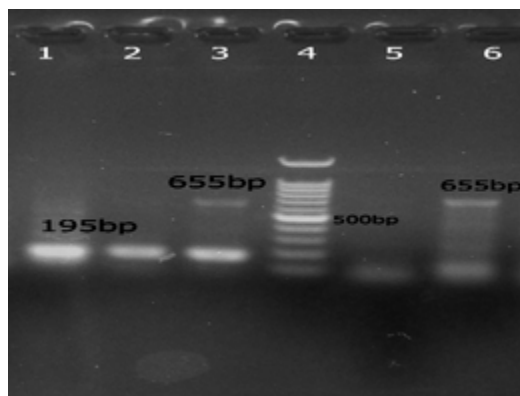
شکل ۳: الکتروفورز محصول PCR دوگانه جستجوی ژن‌های بتا و اپسیلون کلاستریدیوم پرفرینجنس در تعدادی از جدایه‌های کلاستریدیوم پرفرینجنس.
